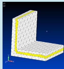
厚さ方向のメッシュ階層
