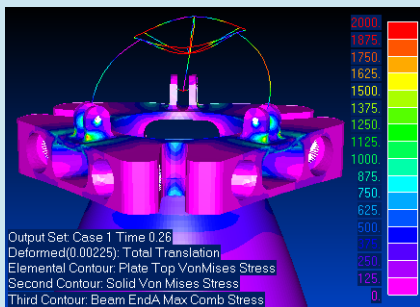
ソリッド、シェル、線要素の結果を同時表示
